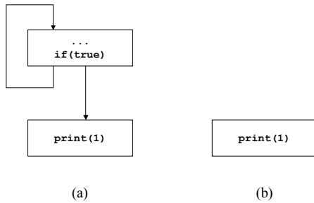
図 6 無限ループの扱い Fig. 6 Handling infinite loop
