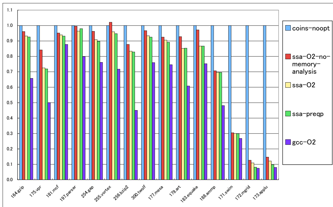
図 10 SPEC ベンチマークによる SSA 最適化器の評価 (COINS 基盤部最適化オプションなしに対する目的コードの実行時間の相対比) Fig. 10 Evaluation of SSA optimizer using SPEC benchmark (ratio of execution time of object code relative to COINS no optimization option)
