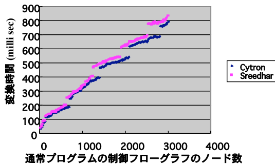
図 4 SSA 変換の変換時間の比較
