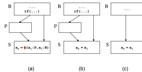
図 8 無用コード除去の望ましい例 Fig. 8 Good example of dead code elimination
