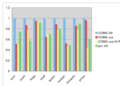
図 11 命令スケジューリング等の適用結果 Fig. 11 Performance after instruction scheduling and others
